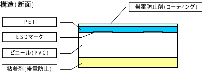
構造(断面)
